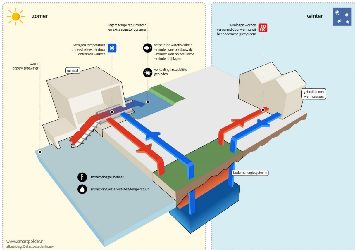
Figuur 1. Werking van TEO met WKO. Bron: Smart polder by IF Technology
